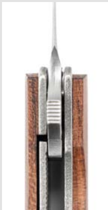
Pos. 7 Die Klinge wird per Kugelhalterung (Detent-Ball) in Position gehalten
